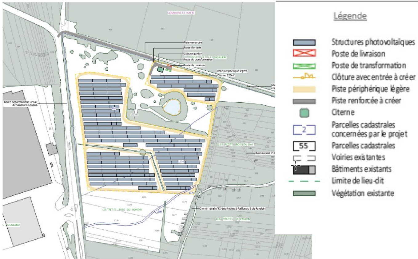
Plan masse du projet – extrait étude d'impact page 20
